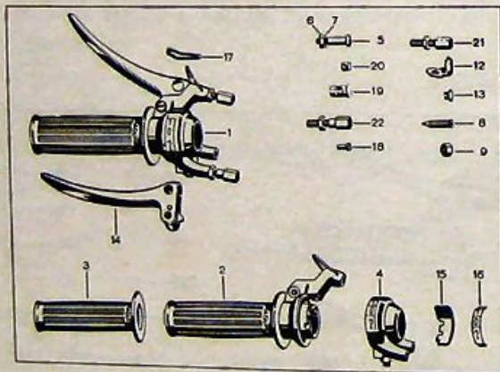
81 934 02 1 Vaihdekädensija, Safir Toimitetaan ainoastaan täyd. kädensijoja
