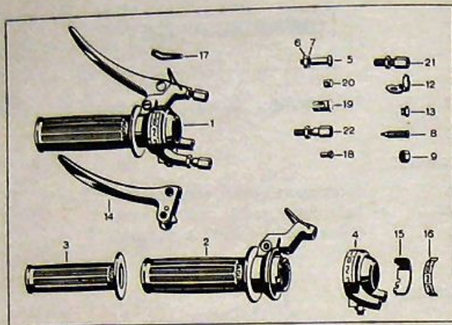
81 933 02 (1) Vaihdekädensija, kädensija rimakuviolla - Sport Toimitetaan ainoastaan täyd. kädensijoja
