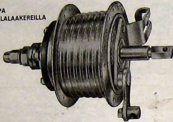
84 650 00 Takanapa pistoakselilla SKF-kuulalaakereilla
