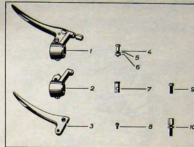
81 940 00 1 Kytinkädensija, jalkavaihte - moottorin, Rally Toimitetaan ainoastaan täyd. kädensijoja
